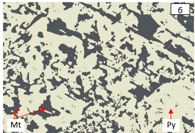
Рис.6. Пирит-магнетитовый агрегат, образующий псевдоморфозу по пирротину. Отраженный свет, без анализатора. а) структуры наблюдаемые в рудах А4; б) структуры, приведенные П. Рамдором, ув. х 250 (Рамдор, 1962).
