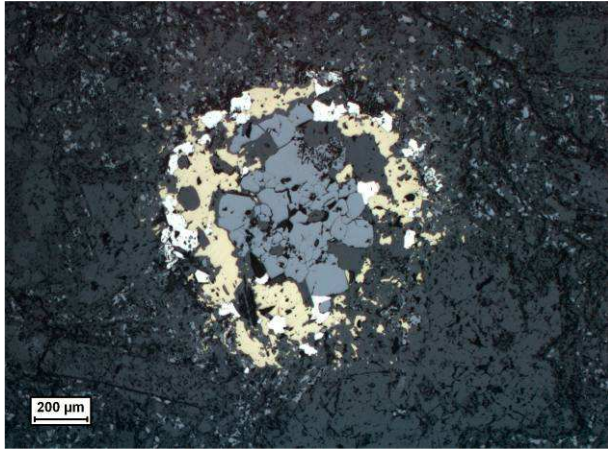
Рис.7. Агрегат рудных минералов, замещающий миндалину андезито-базальта. Оруденелая «миндалина» в скарнированном андезито-базальте с вкрапленностью магнетита. В центре «миндалины» агрегат идиобластовых зерен магнетита, окаймленный халькопиритом с включениями отдельных идиобластовых зерен пирита. Отраженный свет, без анализатора.
