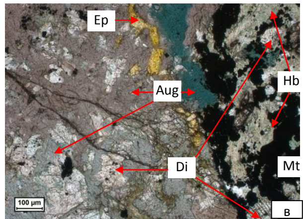
Рис.5. Характер взаимоотношений магнетита в рудах рудопроявления А4. а) сидеронитовая структура сростков магнетита и диопсида. Магнетит формирует грани в сростках с мариалитом. Слабо выраженный идиоморфизм магнетита в сростках с более идиоморфным диопсидом; б) диопсид, находящийся в сростках с магнетитом, в значительной степени замещается роговой обманкой. Мариалит псевдоморфно замещен агрегатом хлорита, полевых шпатов, глинистого минерала и кальцита. Наблюдается корродирование по коротким заливам и трещинам магнетита указанной ассоциацией; в) диопсид замещается двумя минеральными ассоциациями: в левой части снимка эгиринсодержащим авгитом и эпидотом, в правой – преимущественно роговой обманкой и магнетитом; проходящий свет, без анализатора.
